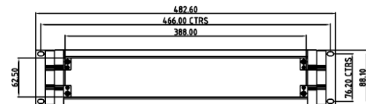
Frontansicht
